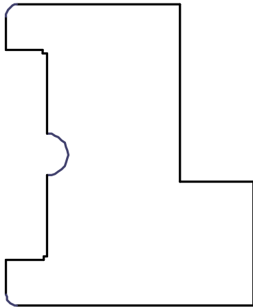
HUISSERIE DE 92 X 60 AVEC CRÂNE SANS CHANFREIN OU BORD DROIT.
