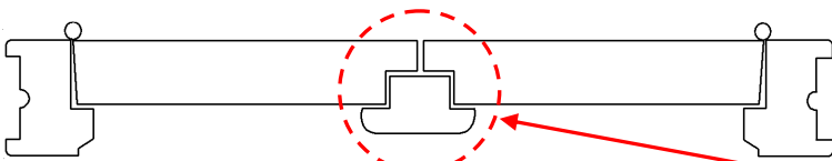
Dimensions hors tout = Largeur de la porte gauche + porte droite + 9 cm d' huisserie Hauteur de la porte + 4.5 cm de traverse.
