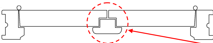
Dimensions hors tout = Largeur de la porte gauche + porte droite + 9 cm d'huisserie Hauteur de la porte + 4.5 cm de traverse.
